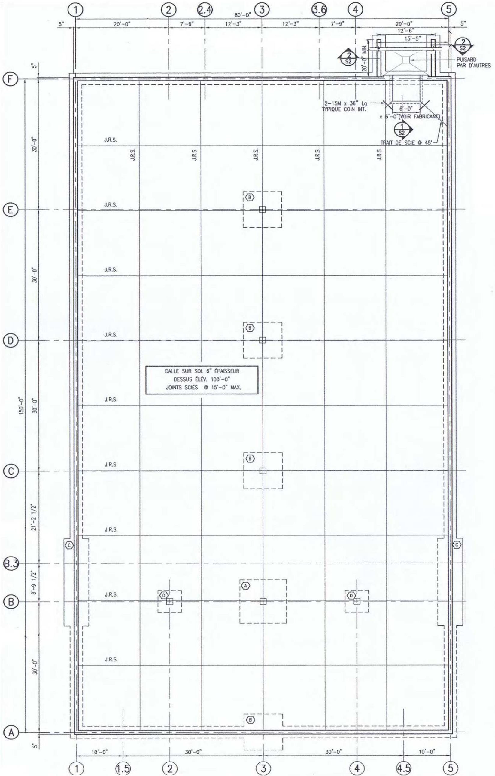
PLAN DES FONDATIONS 14 130, boul. du Curé-Labelle, Mirabel
