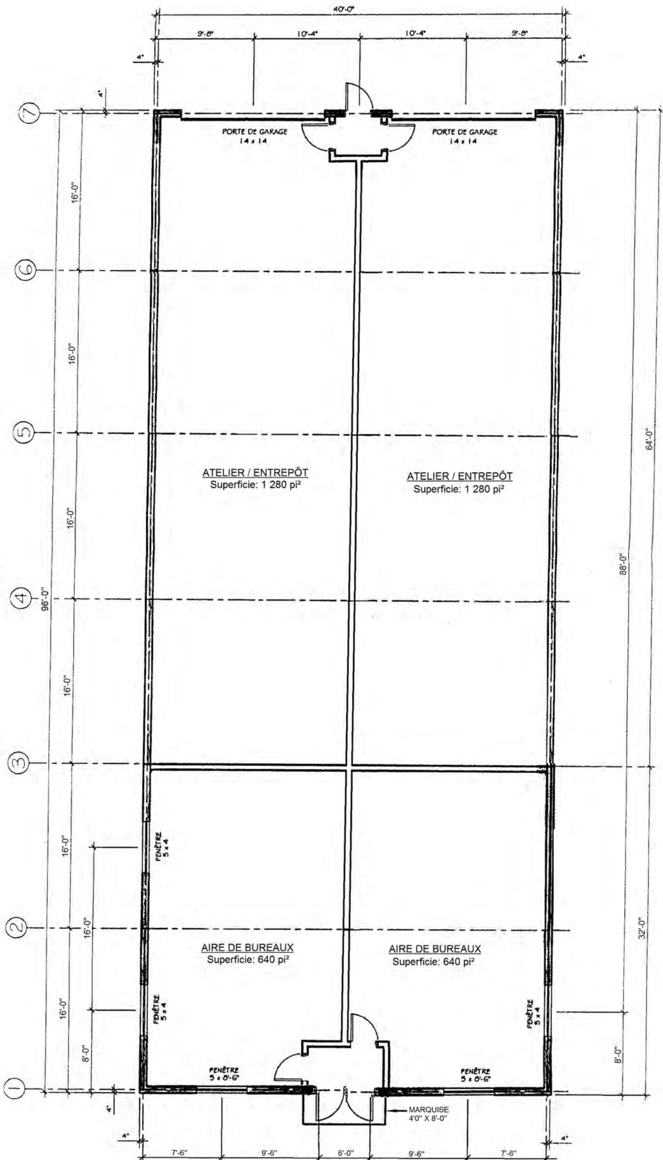
PLAN DU REZ-DE-CHAUSSÉE 14 100, boul. du Curé-Labelle, Mirabel
